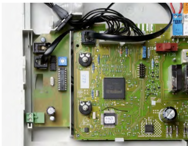
Место установки коммутатора для модулирующих котлов VR 30
